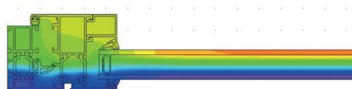
Rozkład temperatur
