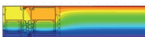
Rozkład temperatur
